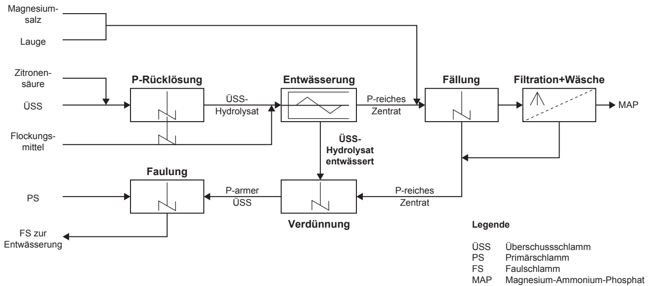
Verfahrensschema des KlimaPhoNds-Verfahrens. © TU Clausthal
