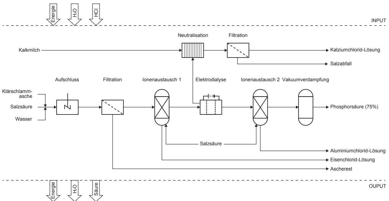
Verfahrensfließschema des AMPHORE-Verfahrens. © Ruhrverband
