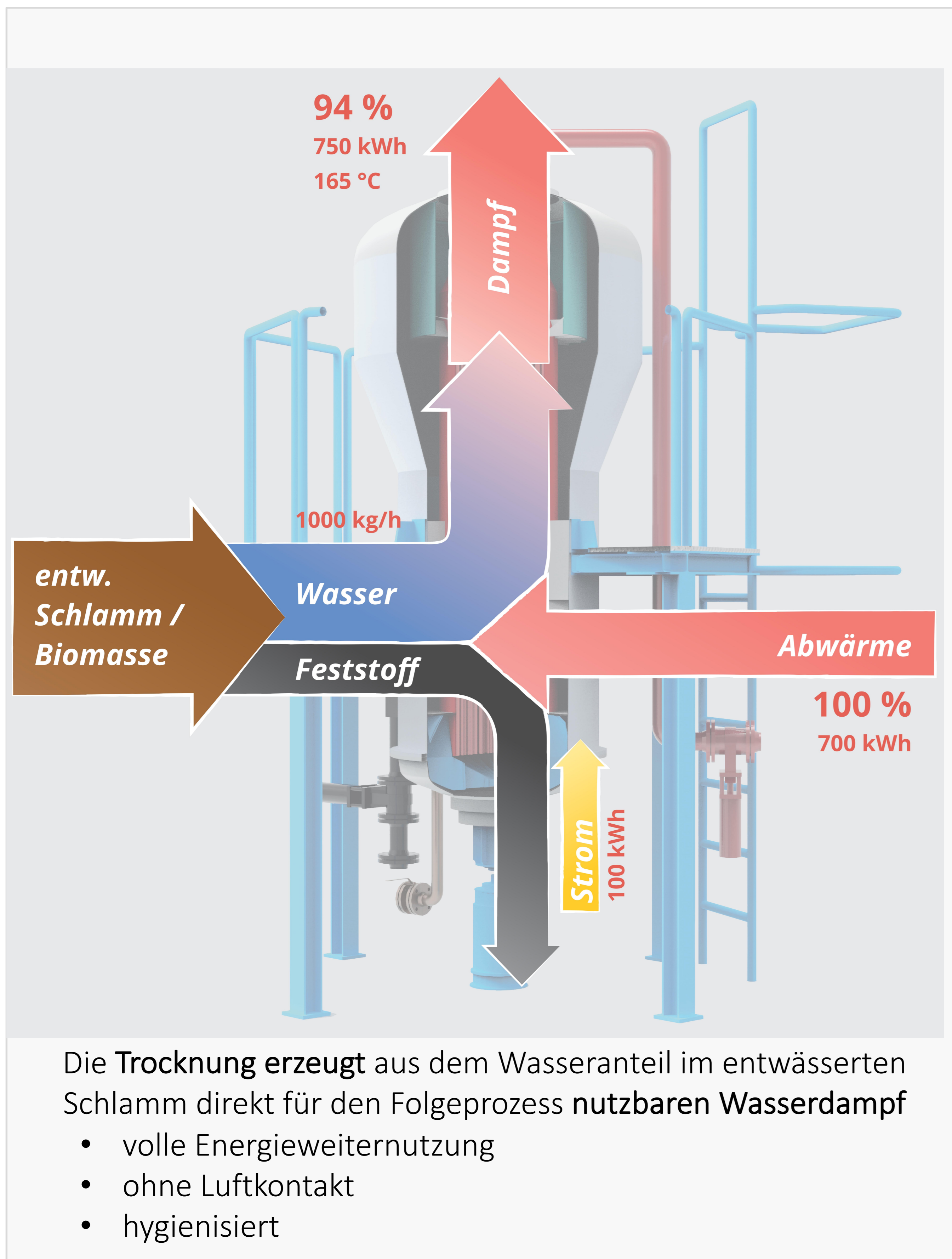
Funktionsschema WWT mit Dampfnutzung
