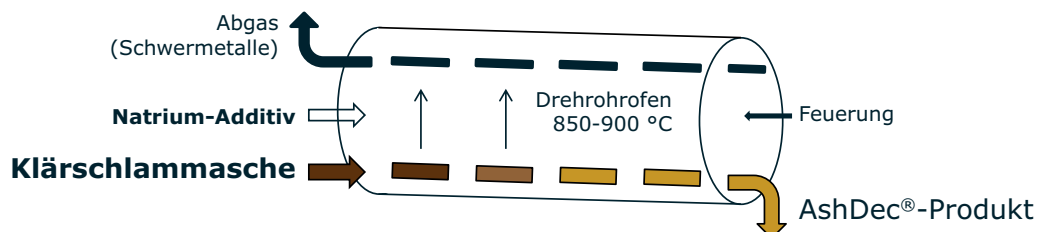
Schema des AshDec®-Prozesses im Drehrohrofen
